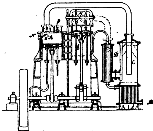
Фиг. 3. Воздушная машина С—ъ Обера.
